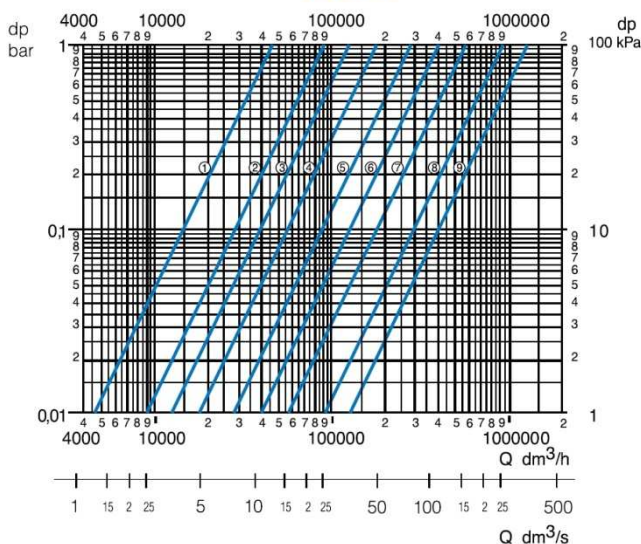
DN300
