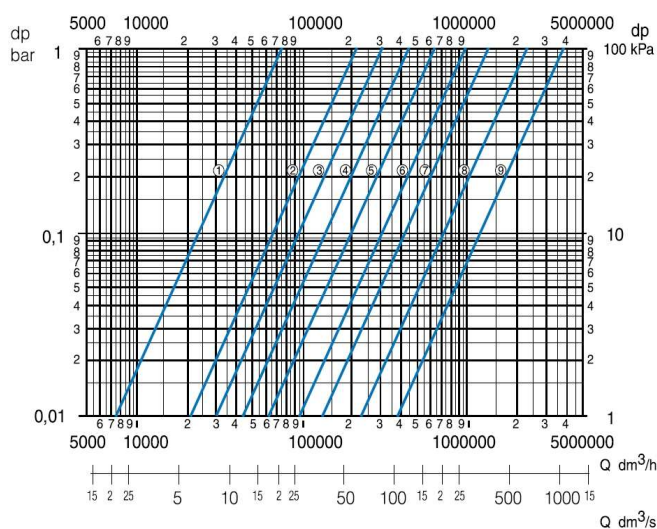
DN300
