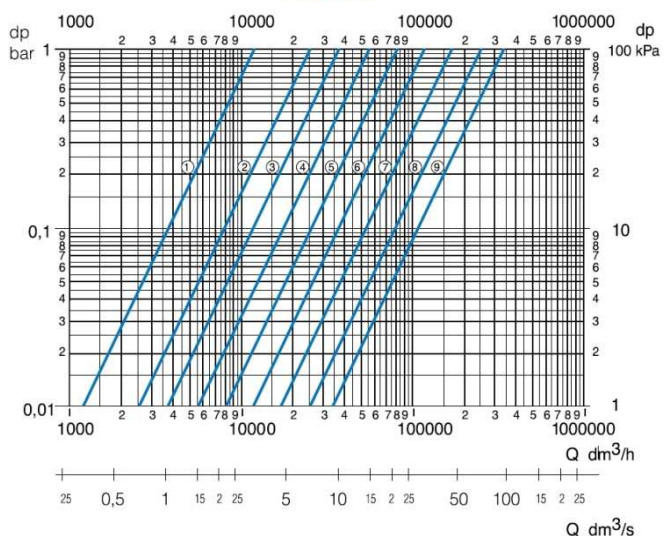
DN150
